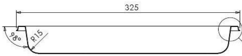
SEZIONE A-A
