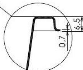
DETTAGLIO
