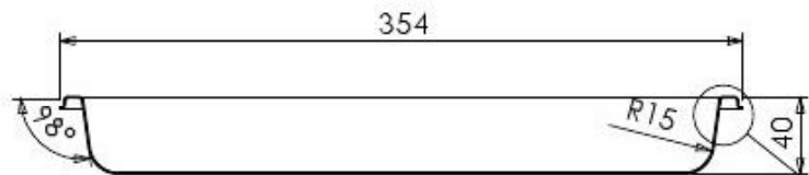
SEZIONE A-A
